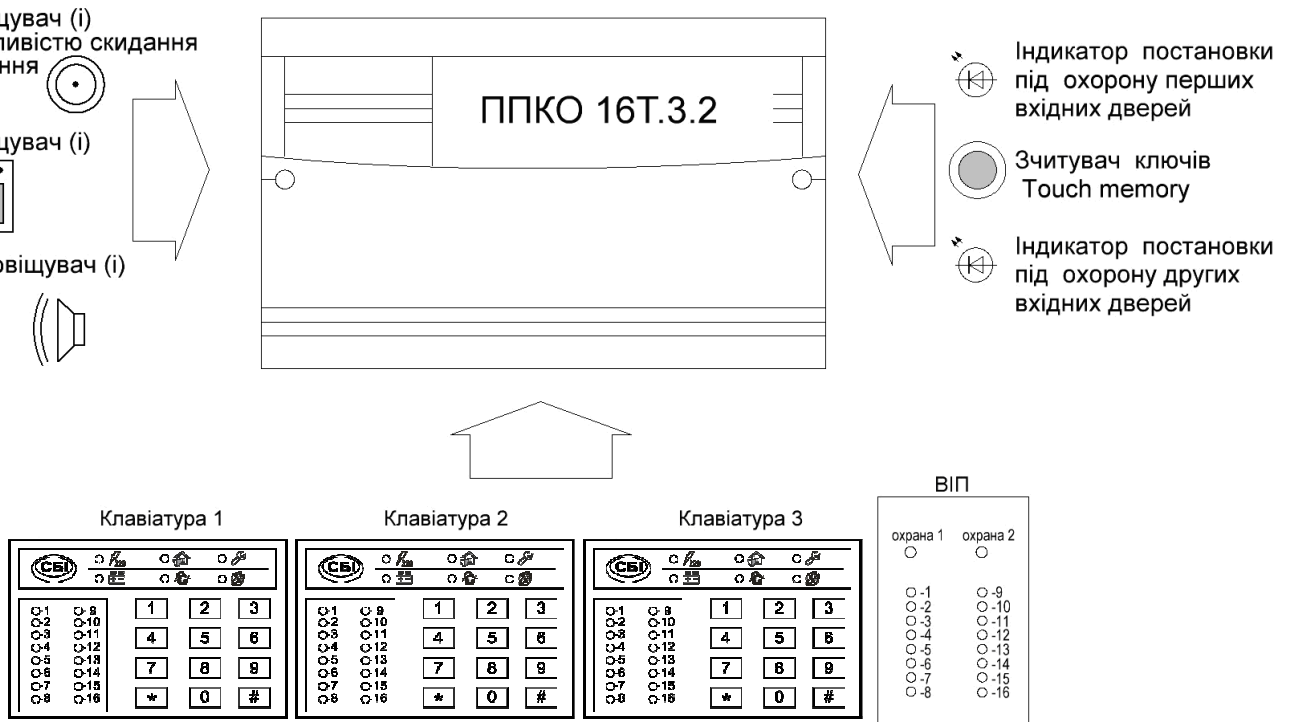
Рисунок 1 – ППКО «Оріон-16Т.3.2 в повному складі.
